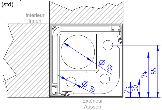
Grondanker Ground anchor Pied fixe à enterrer Grundanker
